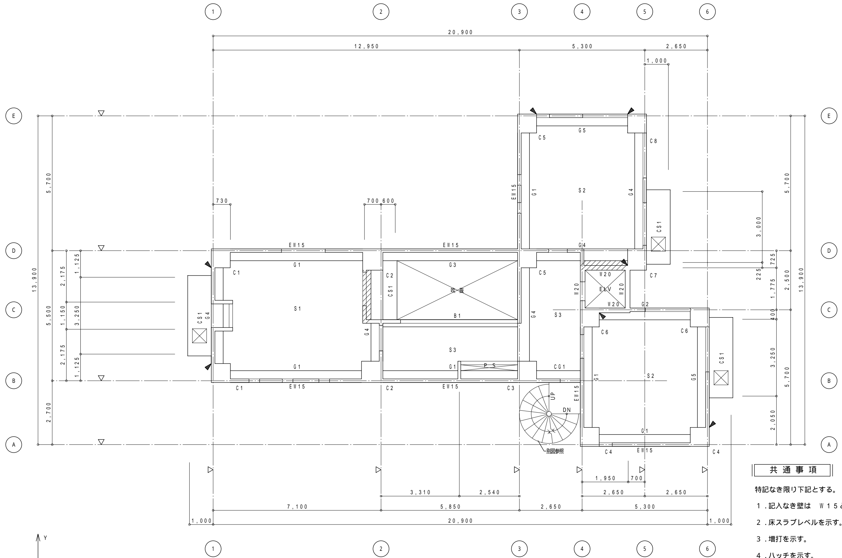
2階壁3階伏図 S=1:100
